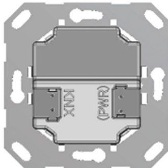
u::Lux NetLink KNX TP – Ansicht von hinten
